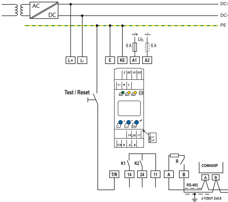
Abbildung: Anschlussbild
